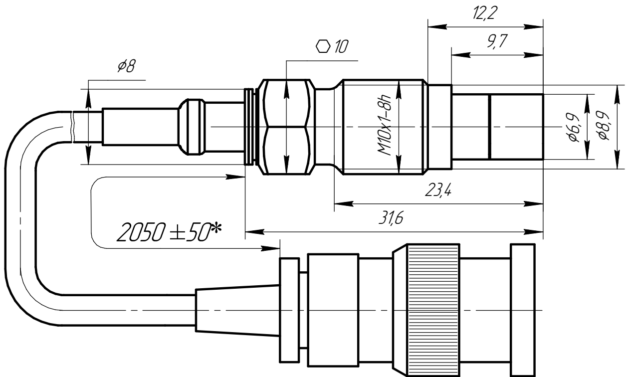
Рис. 2 - АБКЖ.433643.003-01 ГЧ
