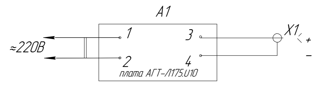
Схема электрическая соединений
